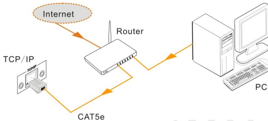
图 5- 4 接入局域网
