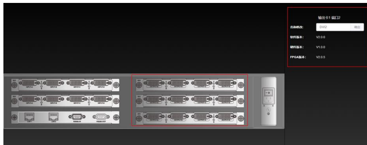
图 8-6 设备输出口配置
