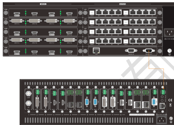
图 4-3 控制第三方设备连接图
