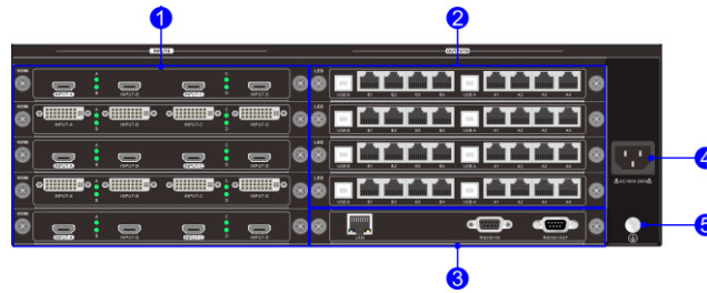
图2-2 后面板
