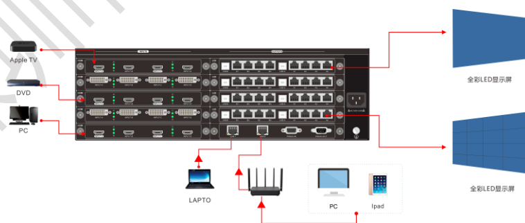
图 4-1 系统连接示意图
